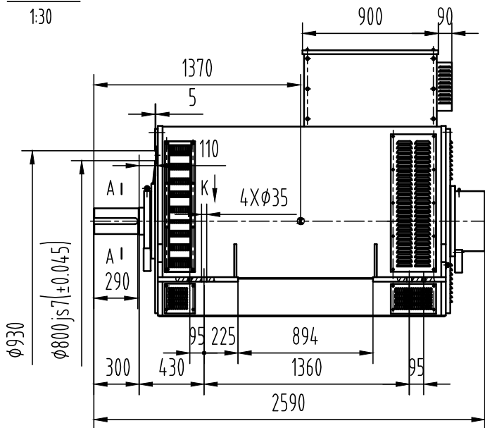
外形安装图
