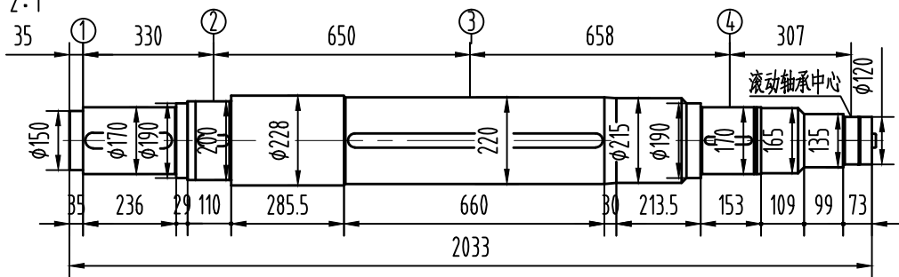
轴系图 2:1
