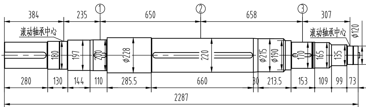
轴系图 2:1
